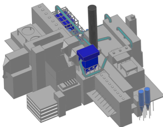
Abbildung 2: Layoutentwurf für eine Verfahrensvariante zur Sanierung der Rauchgasreinigung (Trockenverfahren mit Bicarbonat)
