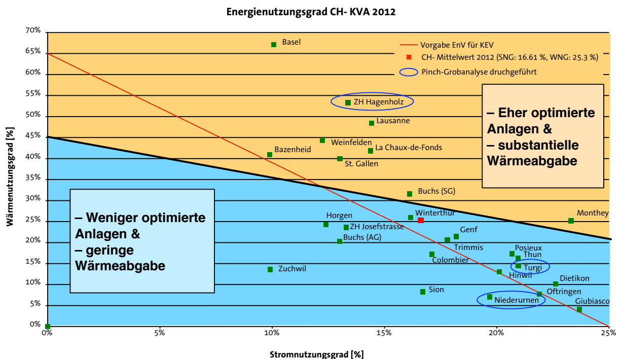
Abbildung 2: Versuch einer groben Gruppierung der Anlagentypen aufgrund ihrer unterschiedlichen Effizienzsteigerungspotentiale wie sie in den Grobanalysen der blau eingekreisten Anlagen gefunden wurden (KVA Linthgebiet = Niederurnen, Grundlagengrafik: BAFU, BFE, Rytec, 2013)
