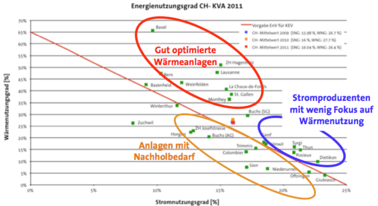
Abbildung 1: Aufteilung der Schweizer KVA in 3 Cluster von Anlagen mit unterschiedlichen Energiesituationen
